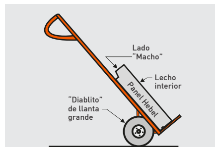
Fig. 6: Posición del panel durante el transporte.
