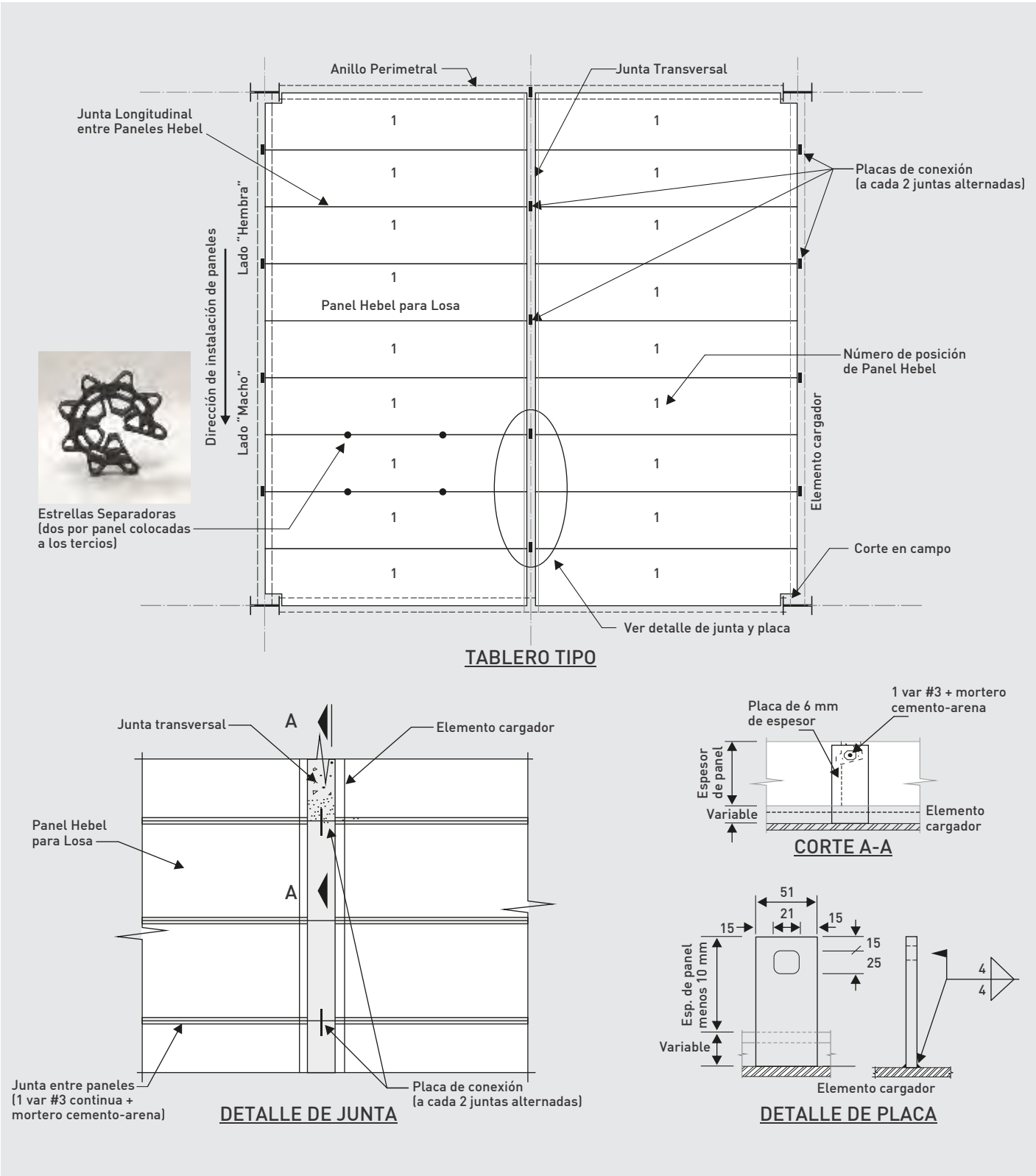
Fig. 12: Tablero tipo de apoyo de paneles sobre estructura de acero.
