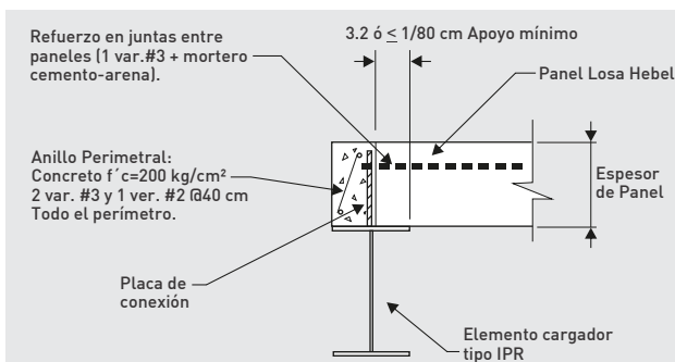
Fig. 18: Detalle de anillo perimetral en elemento de acero.
