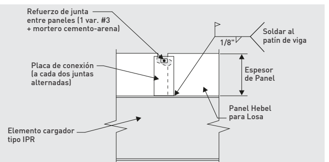
Fig. 17: Placa de conexión en panel Hebel en volado.
