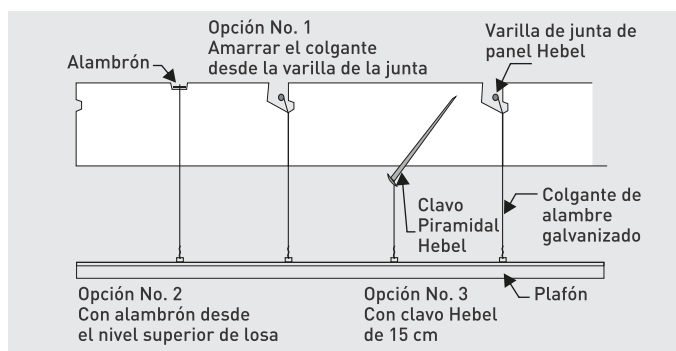
Fig. 26: Colocación de plafón.
