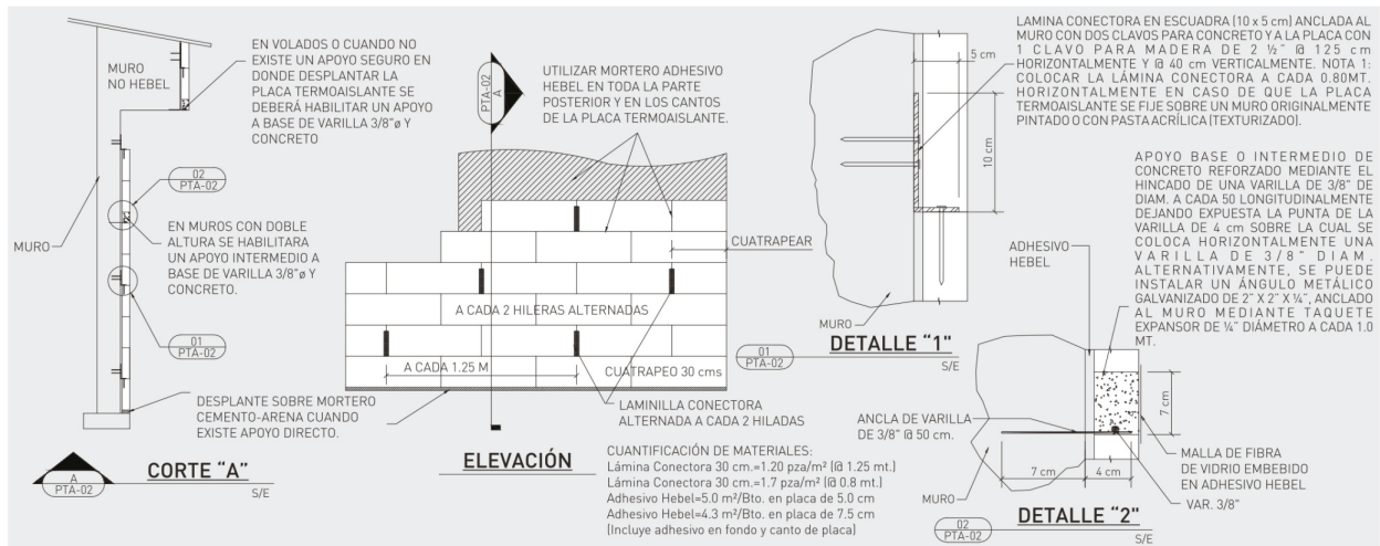
Fig. 2: Placa termoaislante en muro.
