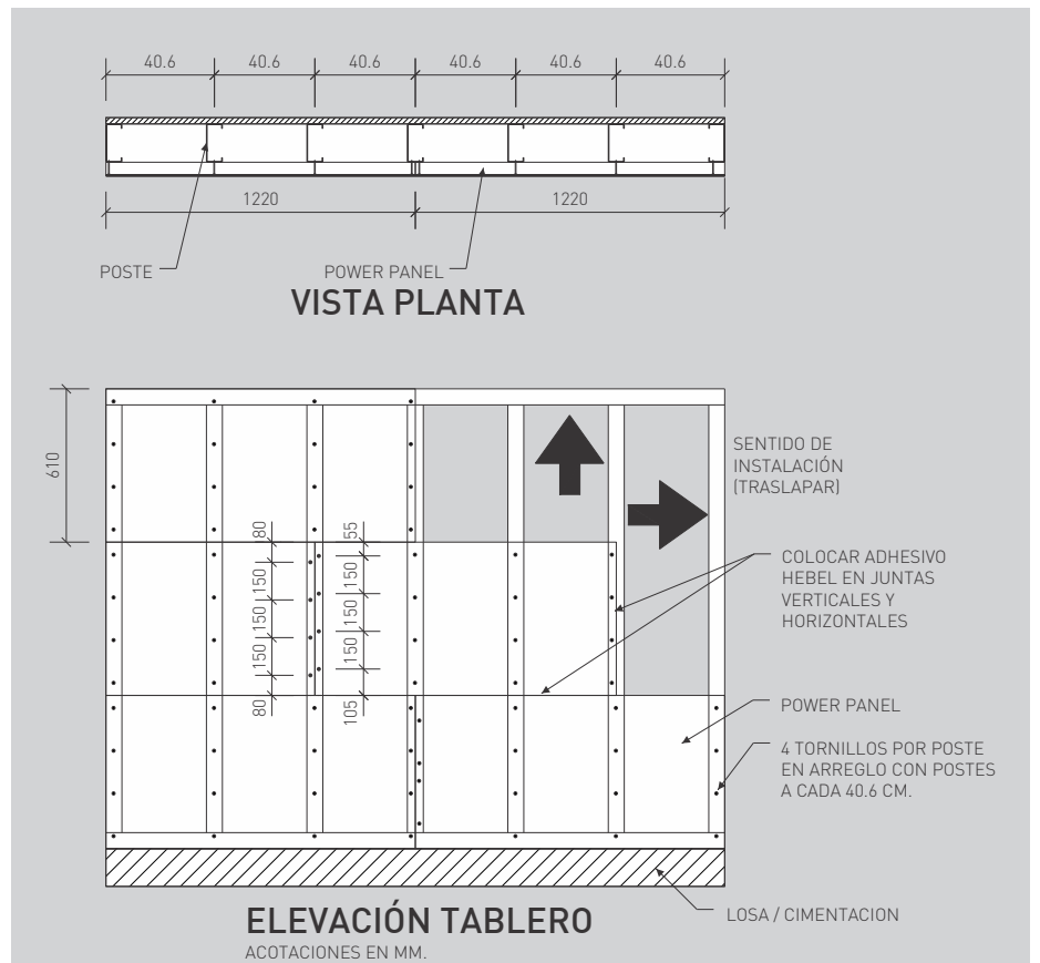
Fig. 15 Distribución de tornillos para fijar Hebel® Power Panel al bastidor metálico.
