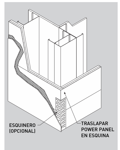
Fig. 20 Detalle de esquina.
