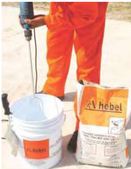
Fig. 7 Preparación de Adhesivo Hebel®.
