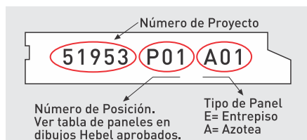
Fig. 2 Identificación de Panel Hebel para Losa.
