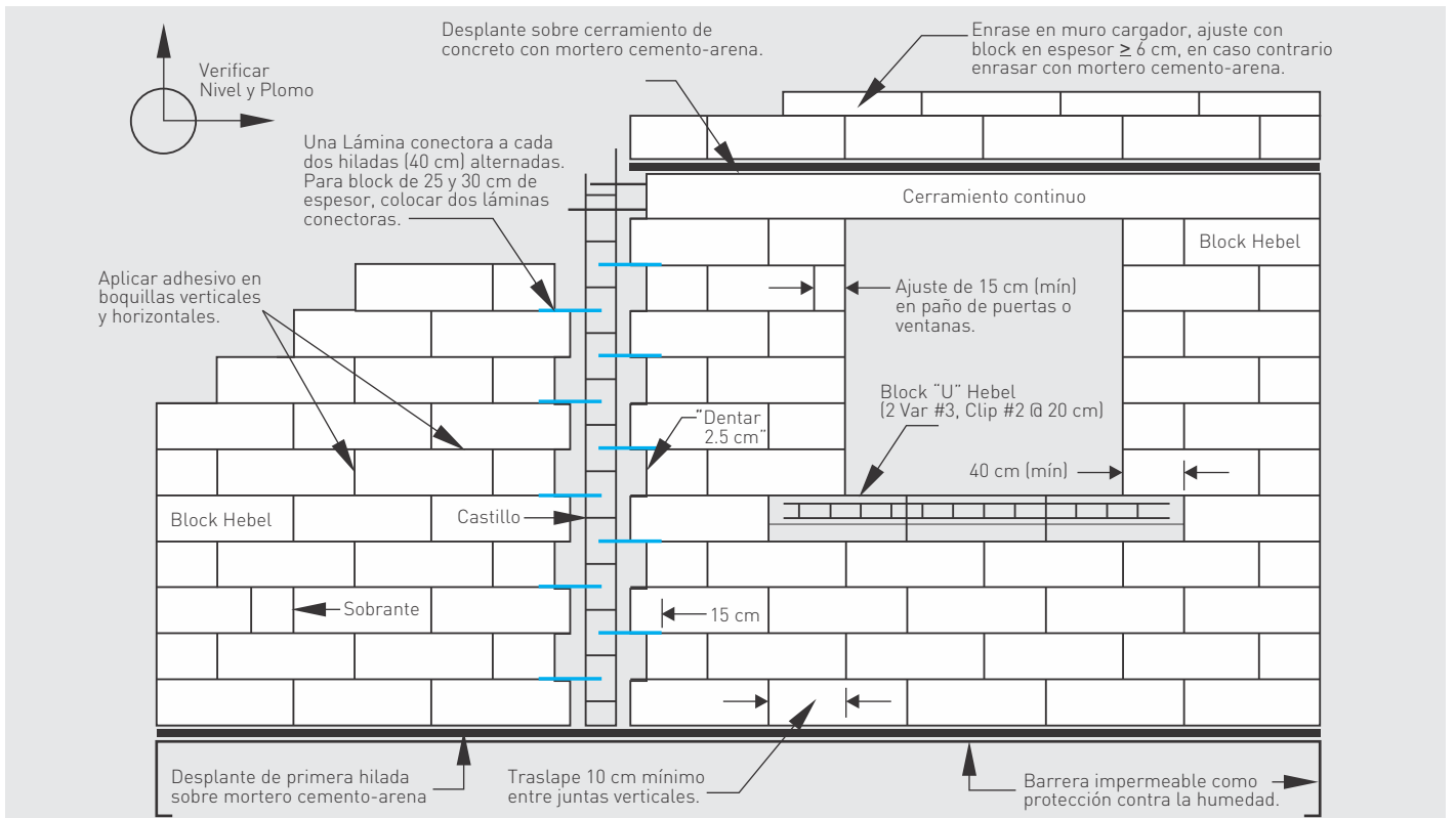
Fig. 12: Detalles constructivos para una correcta instalación de block Hebel.
