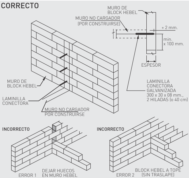
Fig. 13: Unión de muros cargadores a no cargadores.
